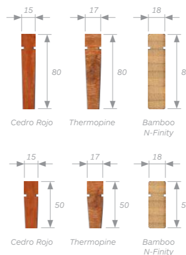
Sección lamas (cotas en mm)
