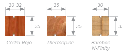
Sección lama (cotas en mm)
